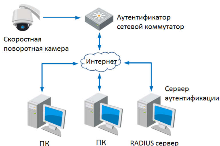
Рисунок 6-20 Защищенная LAN
